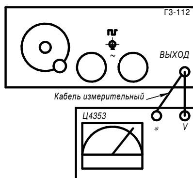
Рисунок 1 - Схема измерения напряжения синусоидального сигнала
